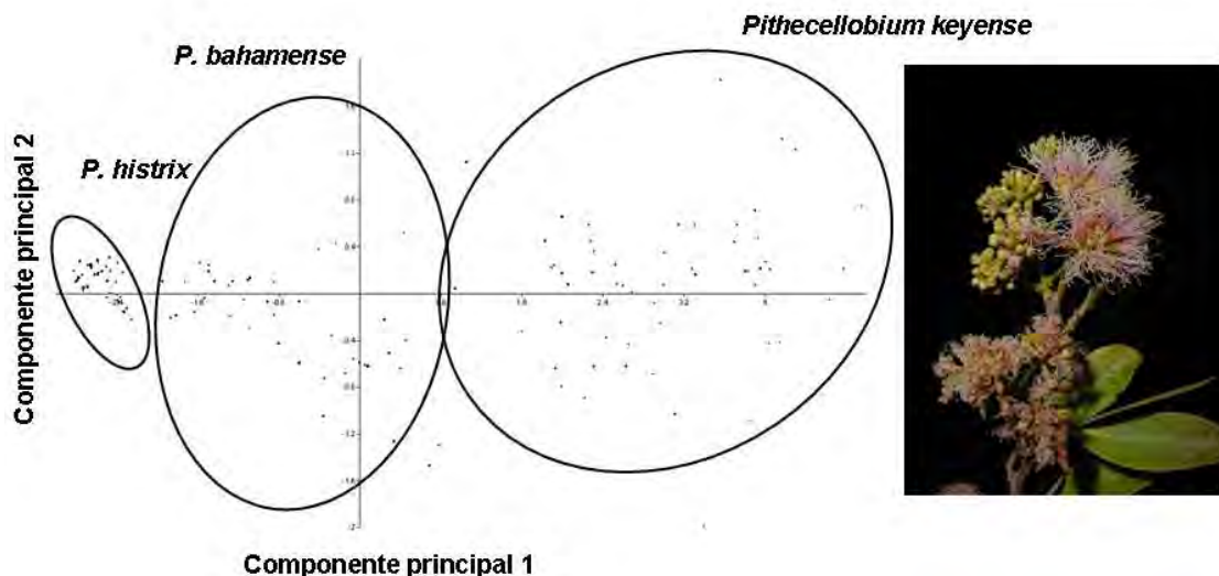
FIGURA 1. Representación gráfica de los datos (especímenes) en el Componente Principal I y Componente principal II. Los dos primeros componentes explican el 98% de la variabilidad de los datos e incluyen información de seis variables continuas obtenidas de la morfología vegetativa (estipulas y hojas) de las dos especies parentales y el híbrido putativo (Imagen: R. Duno).
