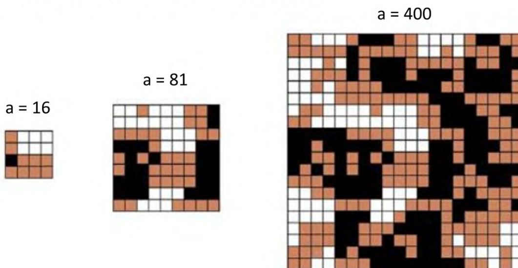
Figura 2. Componentes de la escala. A. grano y B. extensión. (Modificado de Turner et. al. 2001).
