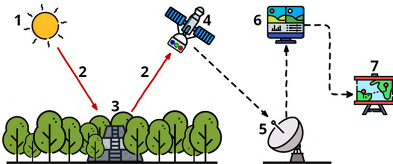
Figura 2. Identificación de elementos del paisaje por medio de sensores remotos, donde: 1) Fuente de energía, 2) Radiación emitida, 3) Elementos del paisaje, 4) Sensor remoto, 5) Recepción de datos, 6) Análisis, 7) Productos. (Tomado de https://geotecinit.github.io/GISDay2020 ).
