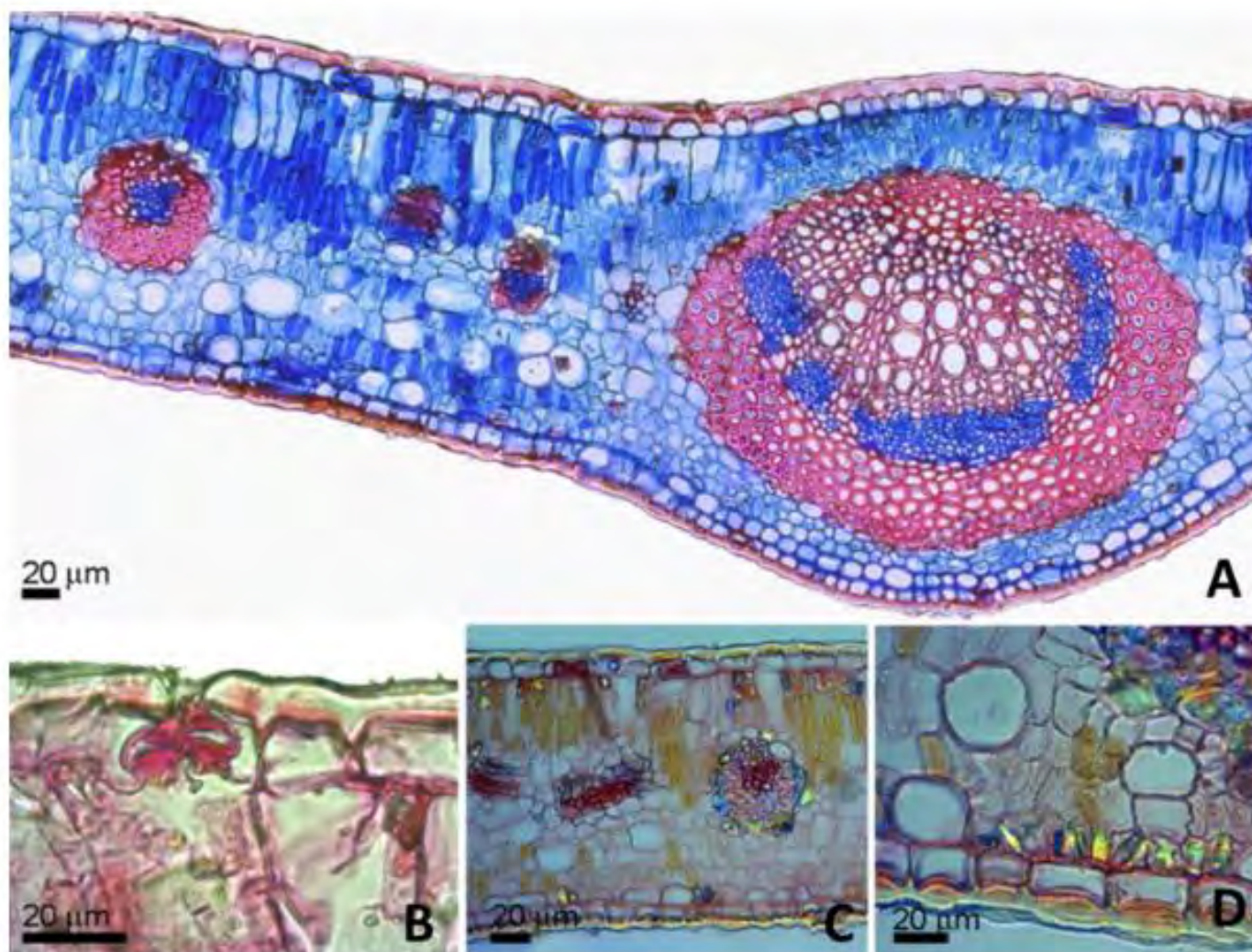
Figura 2. Complejidad del metabolismo secundario. Localización histoquímica in situ de alcaloides en un corte transversal de una hoja de Prosopis ruscifolia , teñida con safranina azul. (Tomado de Gómez et al. 2019).
