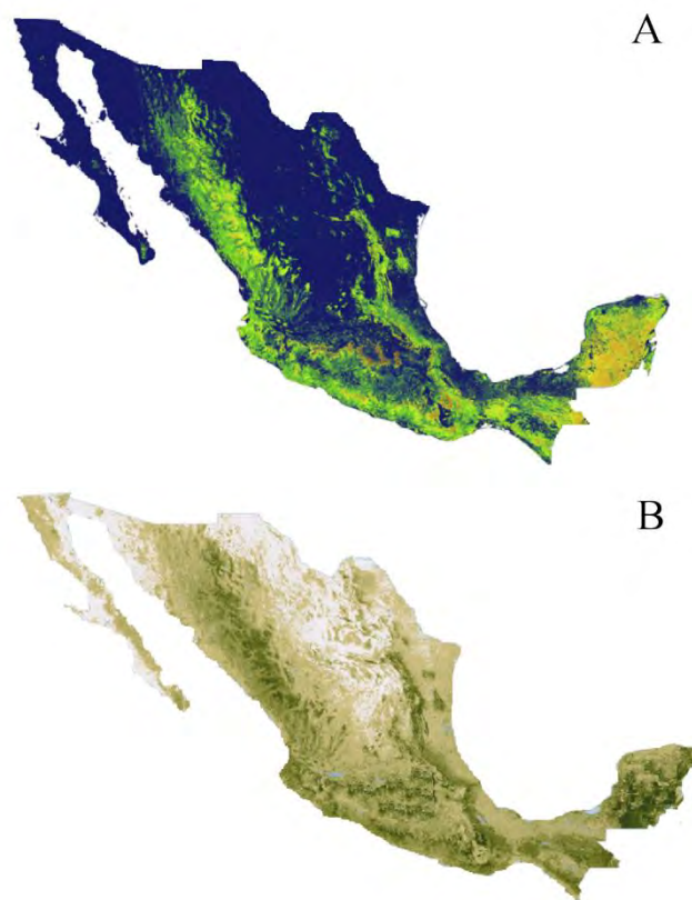
Figura 1. Mapa de México para dos variables. A. Densidad de biomasa aérea (Rodríguez-Veiga et al. 2018) B. Densidad de carbono aéreo (Cartus et al. 2014). Ambos mapas se generaron con datos del Inventario Nacional Forestal, así como variables derivadas de imágenes ópticas (Landsat), de radar (ALOS PAL-SAR), fotografías obtenidas de la misión topográfica de radar (STRM).
