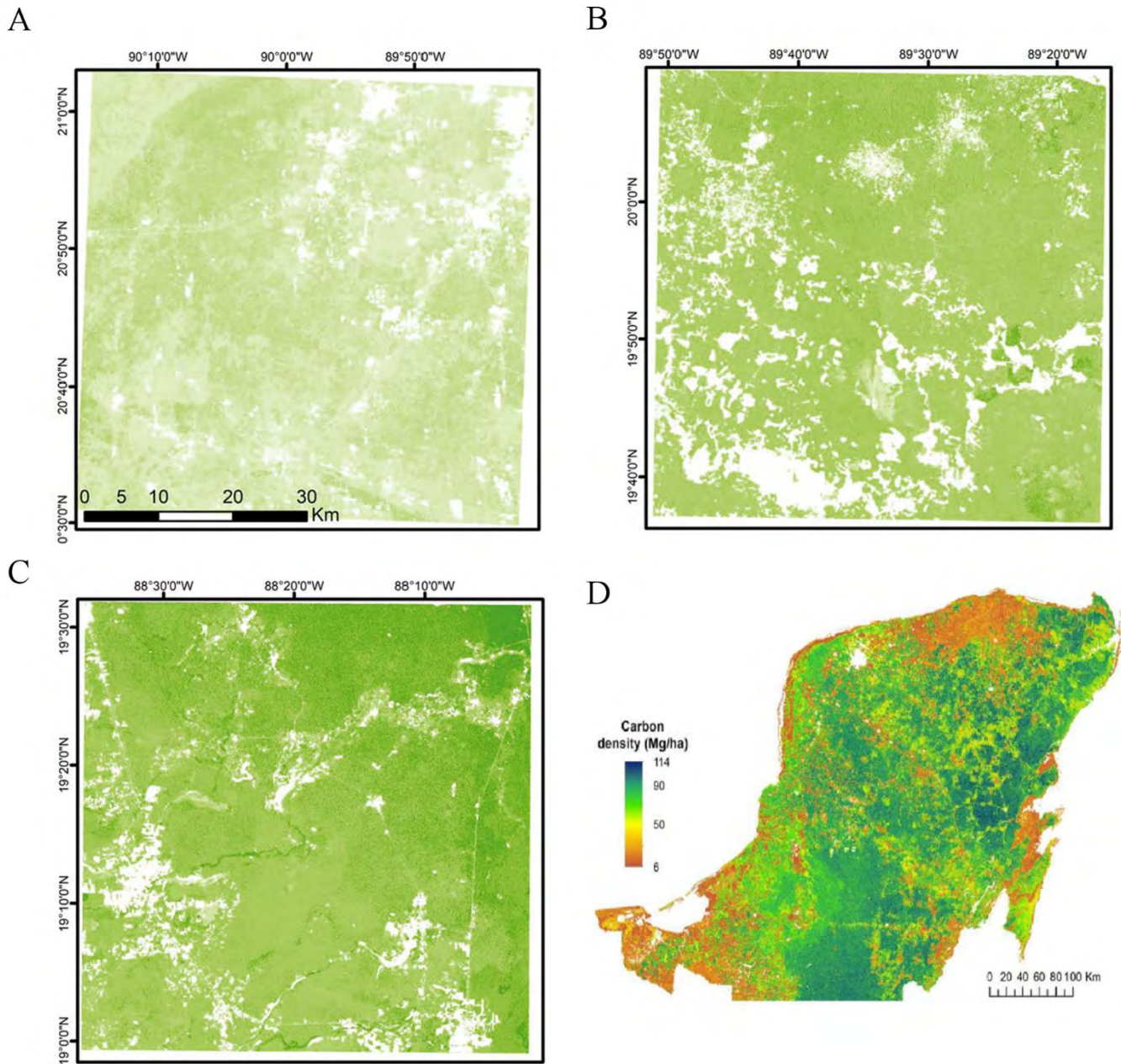
Figura 3. Mapas de densidad de la biomasa aérea. A. Selva caducifolia. B. Selva mediana subcaducifolia. C. Selva mediana subperennifolia. D. Mapa de la densidad de carbono aéreo de la Península de Yucatán. Todos estos mapas se generaron con datos del inventario nacional forestal, así como variables derivadas de imágenes de radar (ALOS PALSAR), y datos de clima, obtenidos en (Hernández-Stefanoni et al. 2020, 2021).
