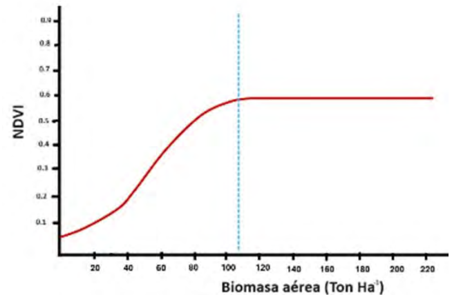
Figura 2. Ejemplificación de la saturación espectral de un índice de vegetación (NDVI=Índice de Vegetación de Diferencia Normalizada). La saturación del índice comienza cuando los valores de biomasa aérea son más grandes (a partir de la línea azul).
